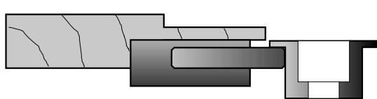
TENON LONG DOUBLE EPAULEMENT EN 2 PASSES
