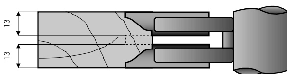
PROFIL DOUBLE PAREMENT
