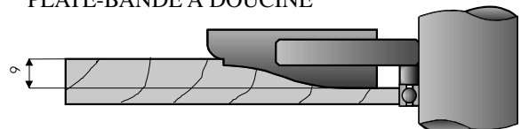
PLATE-BANDE A DOUCINE
