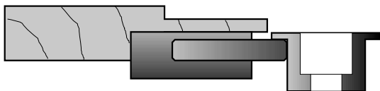
TENON LONG DOUBLE EPAULEMENT EN 2 PASSES
