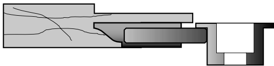
TENON LONG CONTREPROFILE EN 2 PASSES
