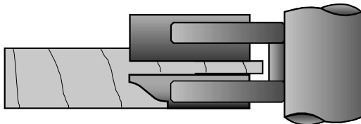
TENON LONG CONTREPROFILE EN 1 PASSE
