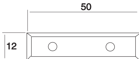
① Fournie avec le Porte-Outil PLAQ0246
